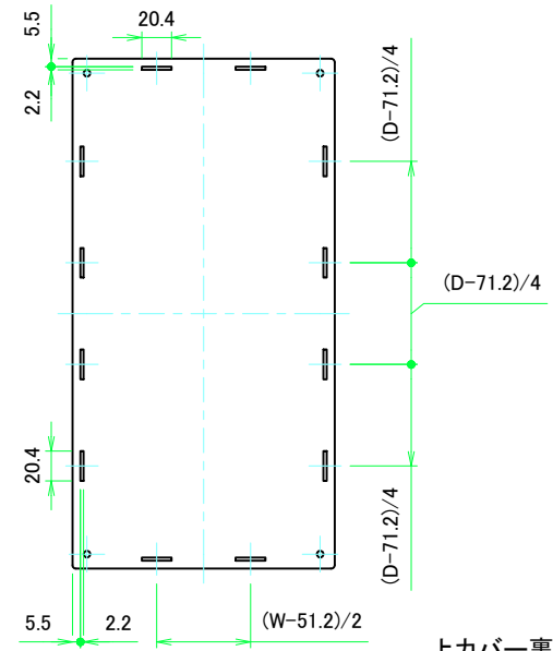
上カバー裏面 / Top cover Backside
