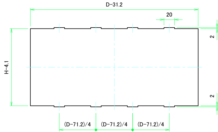
Dパネル1表面 / D Panel 1 Frontside
